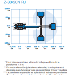
Diagrama de trabajo del plúmin Z-30/20N RJ
