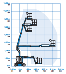
Diagrama de trabajo Z-30/20N RJ
